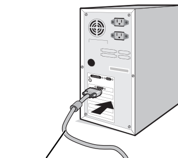
Cavo per segnali mini D-SUB a 15 pin Figura A.2
