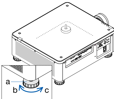
а: Ножка регулировки наклона / b: Вверх / c: Вниз
