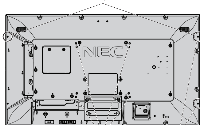
Interfejs montażowy VESA (M6)
