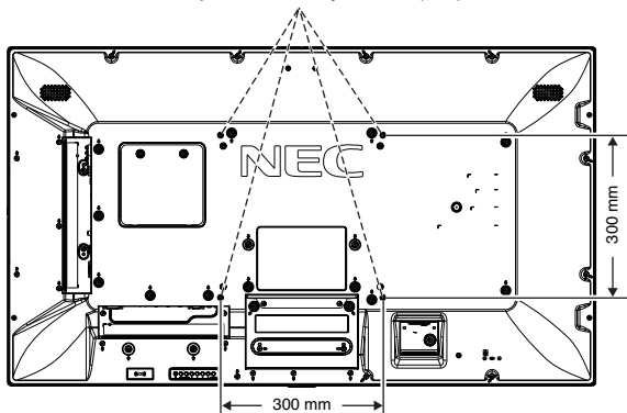
Interfejs montażowy VESA (M6)
