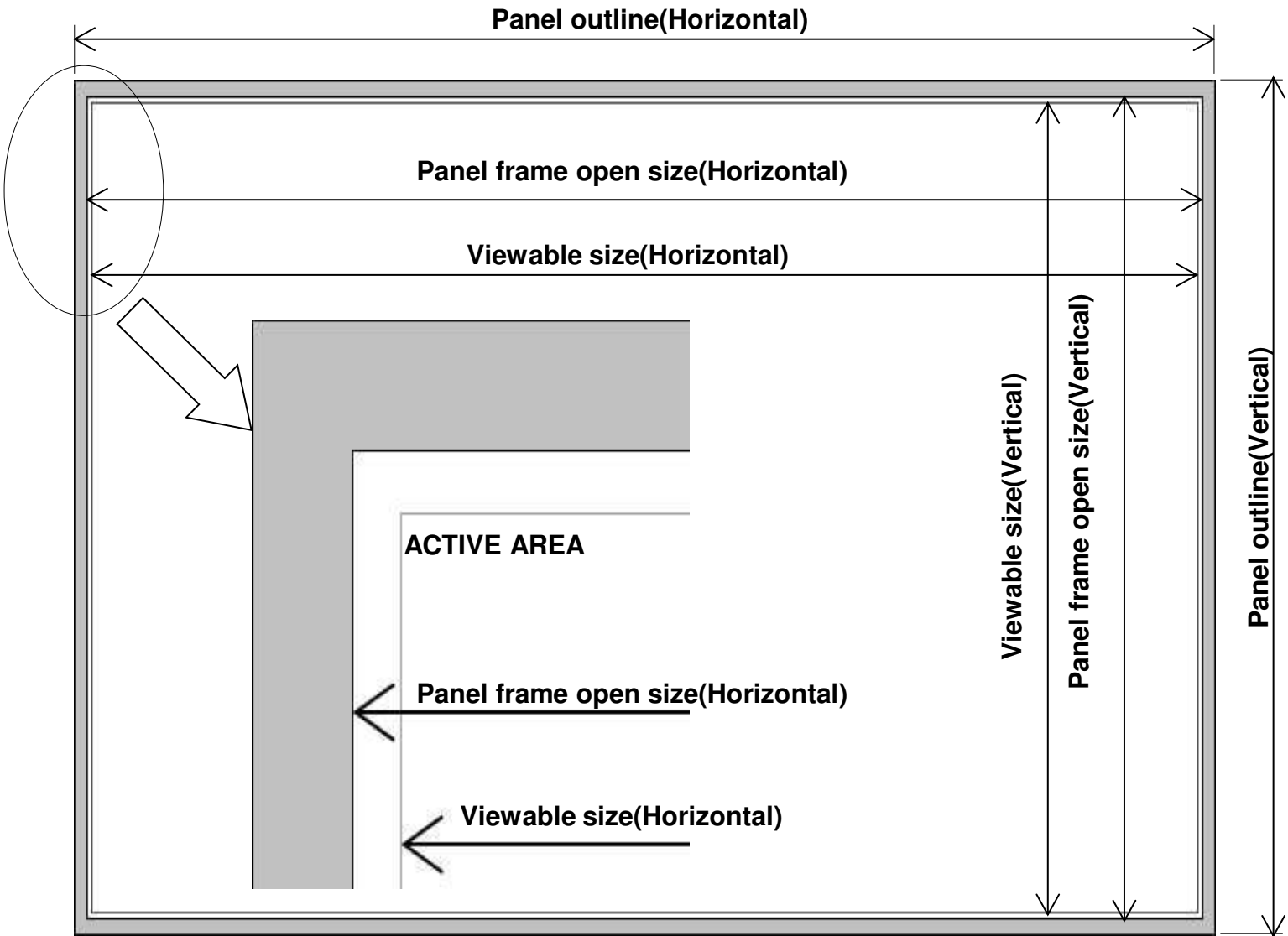
LCD Module
