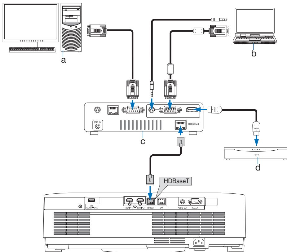
a: Dator (för styrning)/b: Dator (för utmatning)/c: Exempel på en sändarenhet/ d: Enhet för utmatning av HDMI-video
