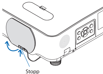
Projektor
