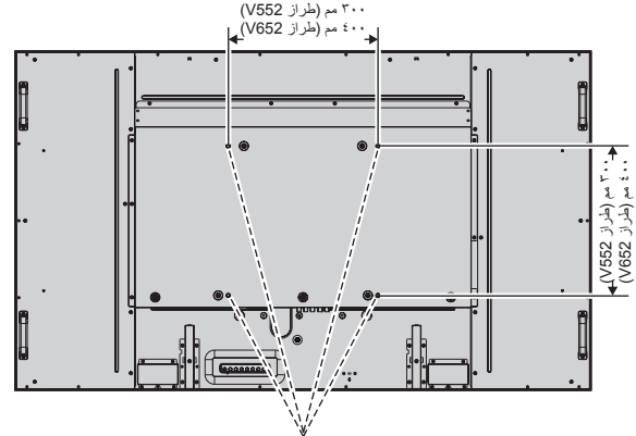
واجهة تثبيت الذراع المتوافقة مع معايير VESA
