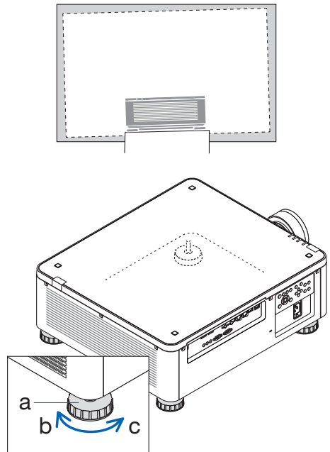
a: Kippfuß / b: Nach oben / c: Nach unten
