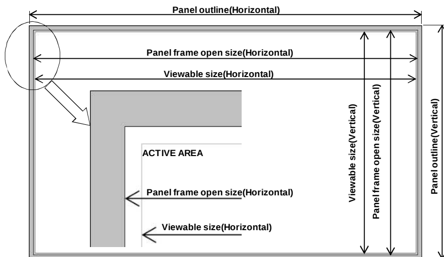
LCD Module
