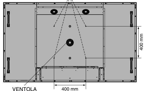
Interfaccia di montaggio VESA
