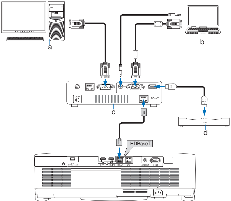
a: Tietokone (ohjauskäyttöön) / b: Tietokone (lähtökäyttöön) / c: Esimerkki lähetinlaitteesta / d: HDMI-lähtövideolaite
