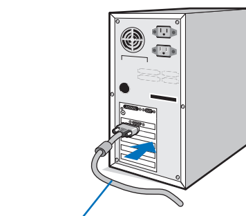
Signalkabel mit 15-poligem Mini-D-SUB-Stecker Abbildung A.3
