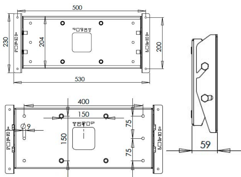
WM-BT - DIMENSIONS
