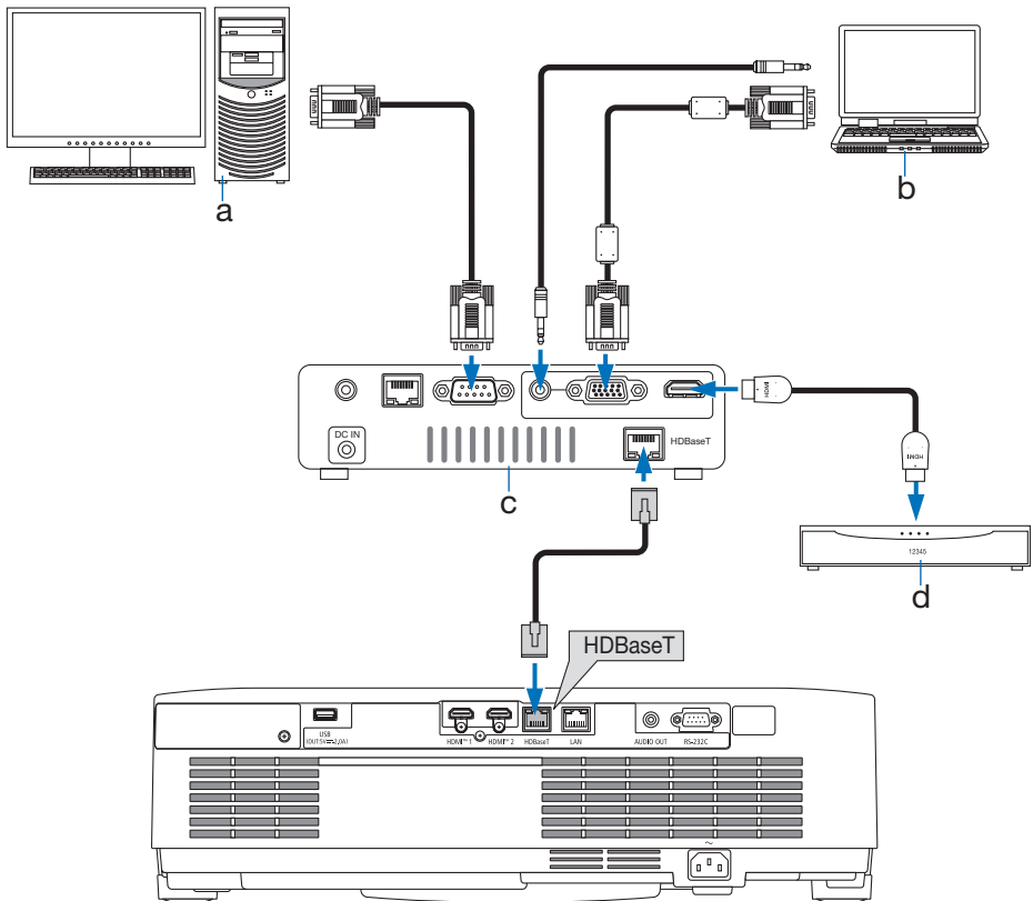
a: Computador (usado para controle) / b: Computador (usado para a saída) / c: Exemplo de um dispositivo de transmissão / d: Dispositivo de vídeo com saída HDMI
