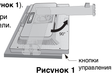
Рисунок 1 кнопки управления
