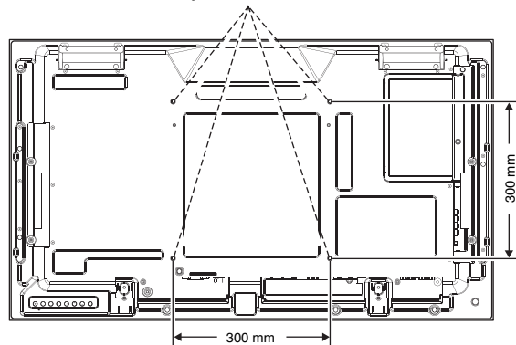
Montážní vybavení standardu VESA
