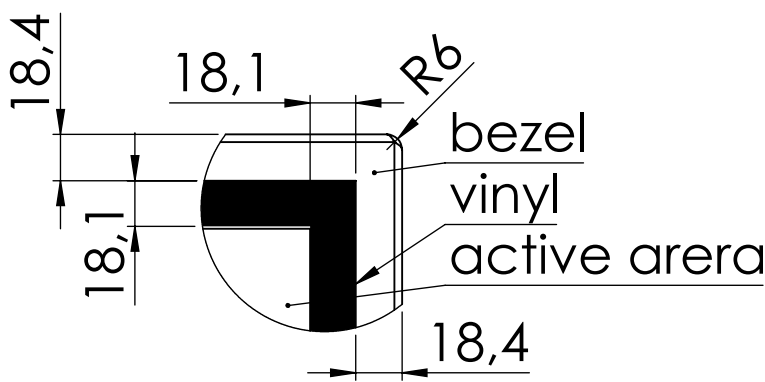
SZCZEGÓŁ A SKALA 1 : 3
