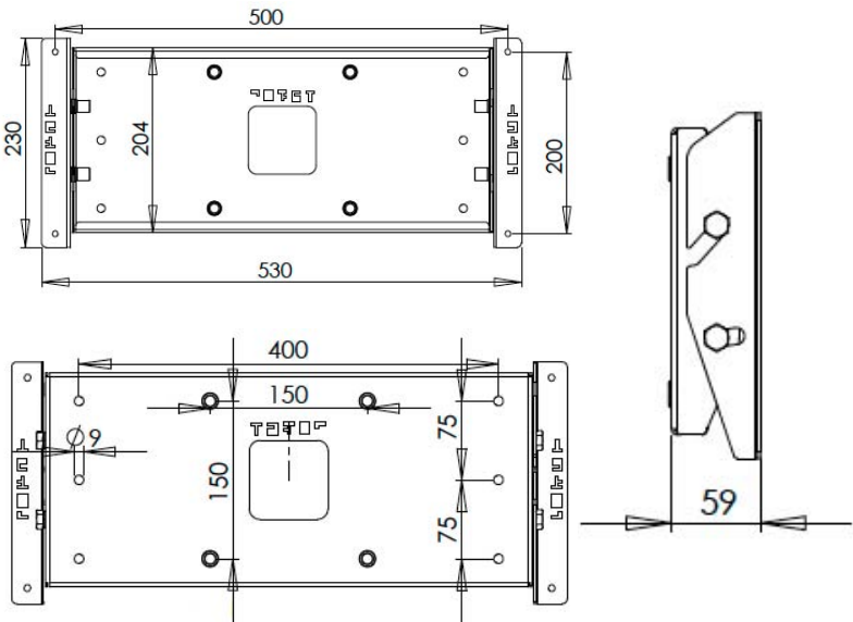
WM-BT - DIMENSIONS
