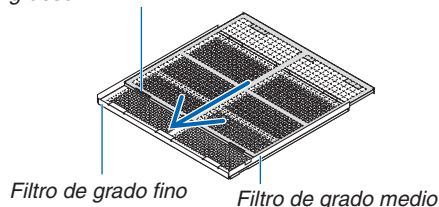
Las ranuras de pestaña en el filtro de grado grueso
